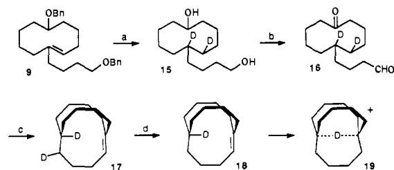
(a) D 2 , Pd/C, CH 3 OH, EtOAc, HOAc; (b) PCC, CH 2 Cl 2 , NaOAc; (c) TiCl 3 (DME) 1.5 , Zn-Cu, DME; (d) HCl, H 2 O.
